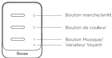
Boîtier de commande
